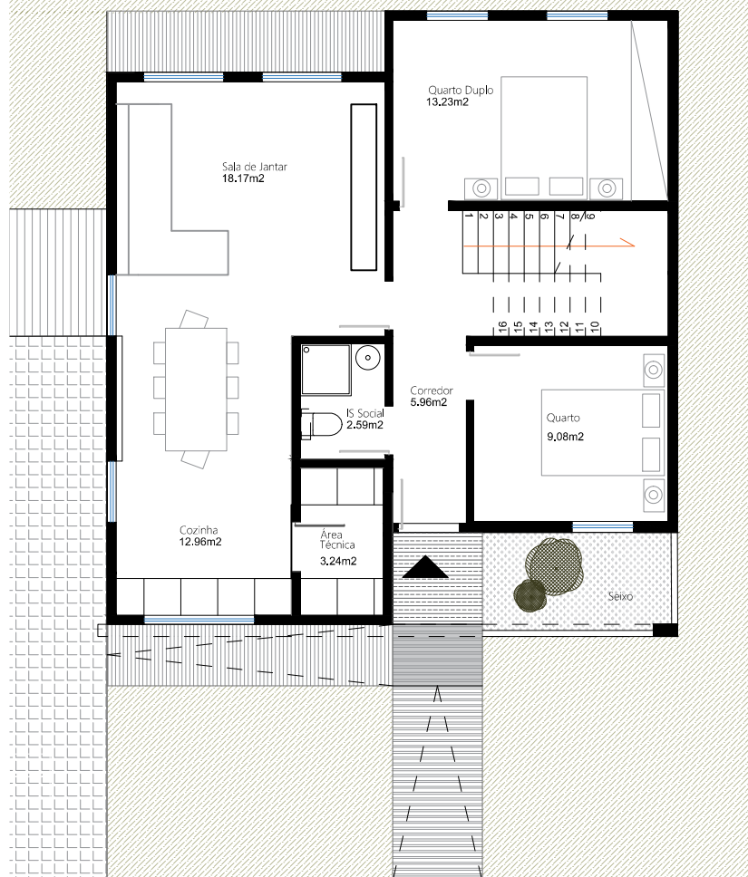
PISO 0
